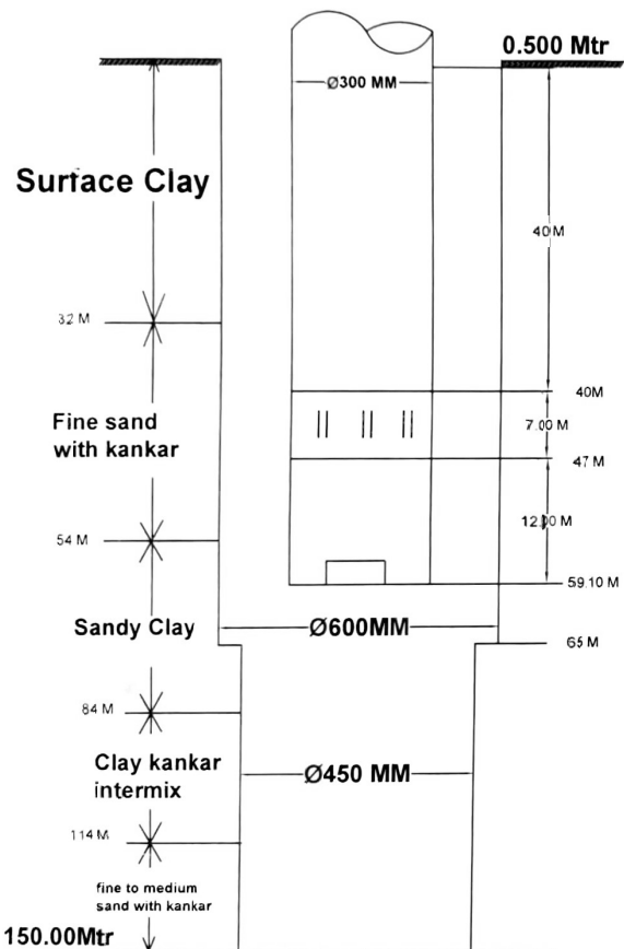
Actual Tubewell Assembly Lowering Chart
