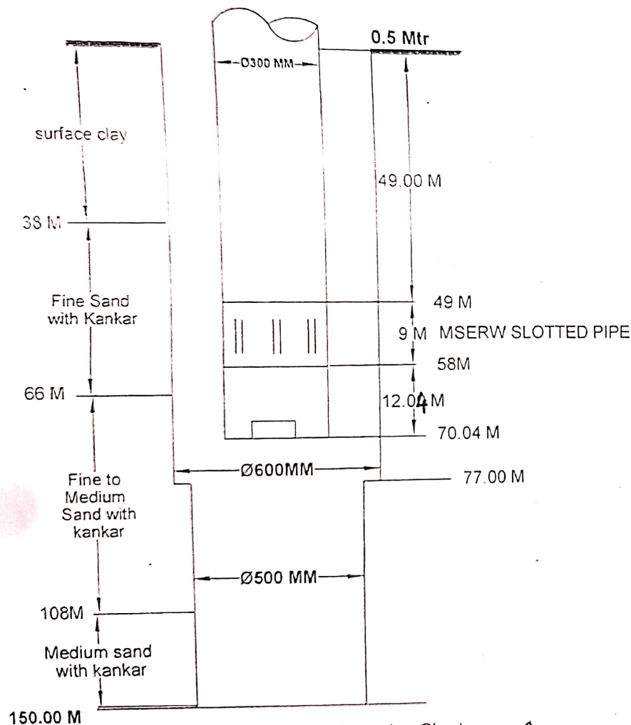
Actual Tubewell Assembly Lowering Chart
